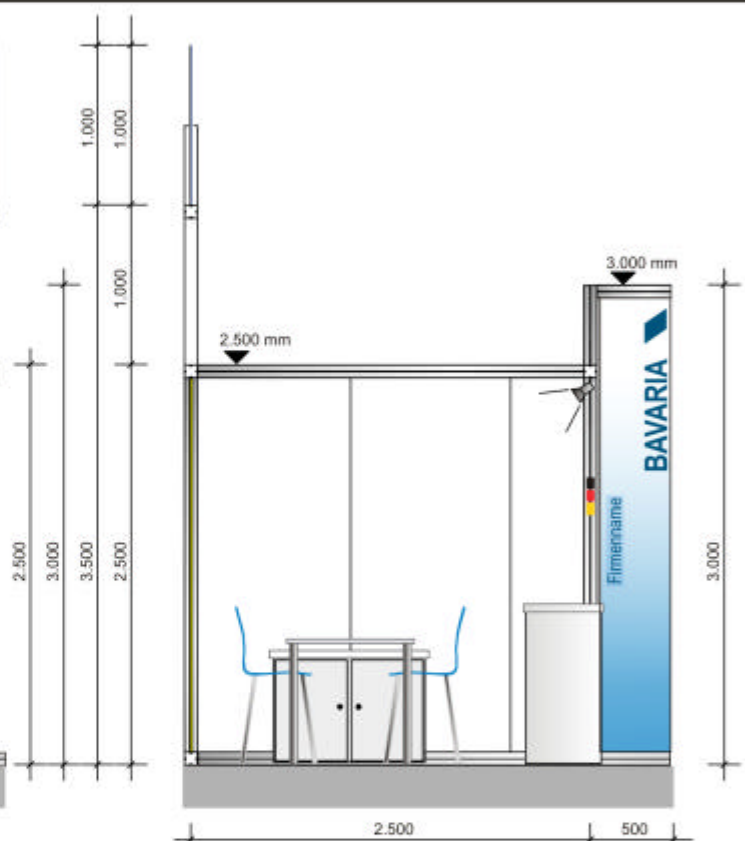
Schnitt Section
