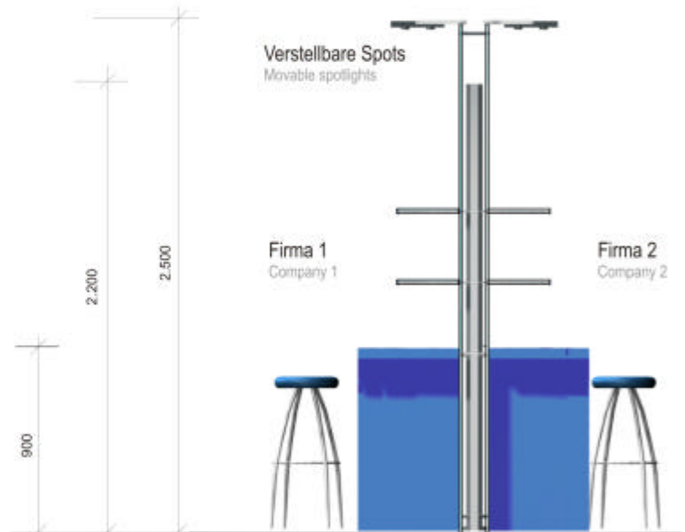
Schnitt Section
